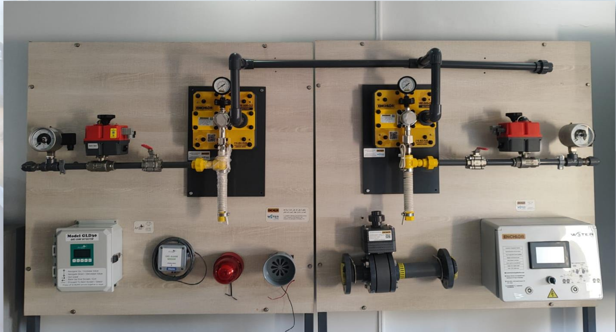
منظومة تحويل اتوماتيكي سعة 40 كجم/س + جهاز انذار بمشتملاته
